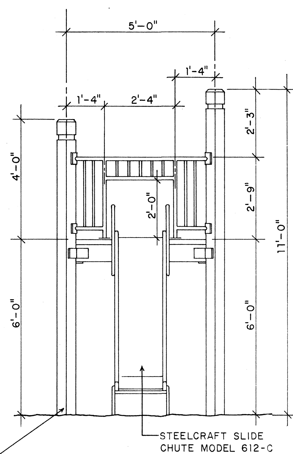
ELEVATION 2
