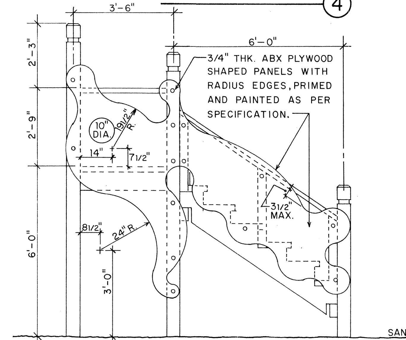
ELEVATION 4
