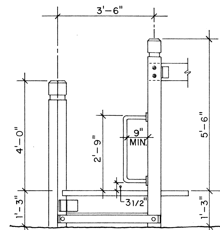
ELEVATION 7
