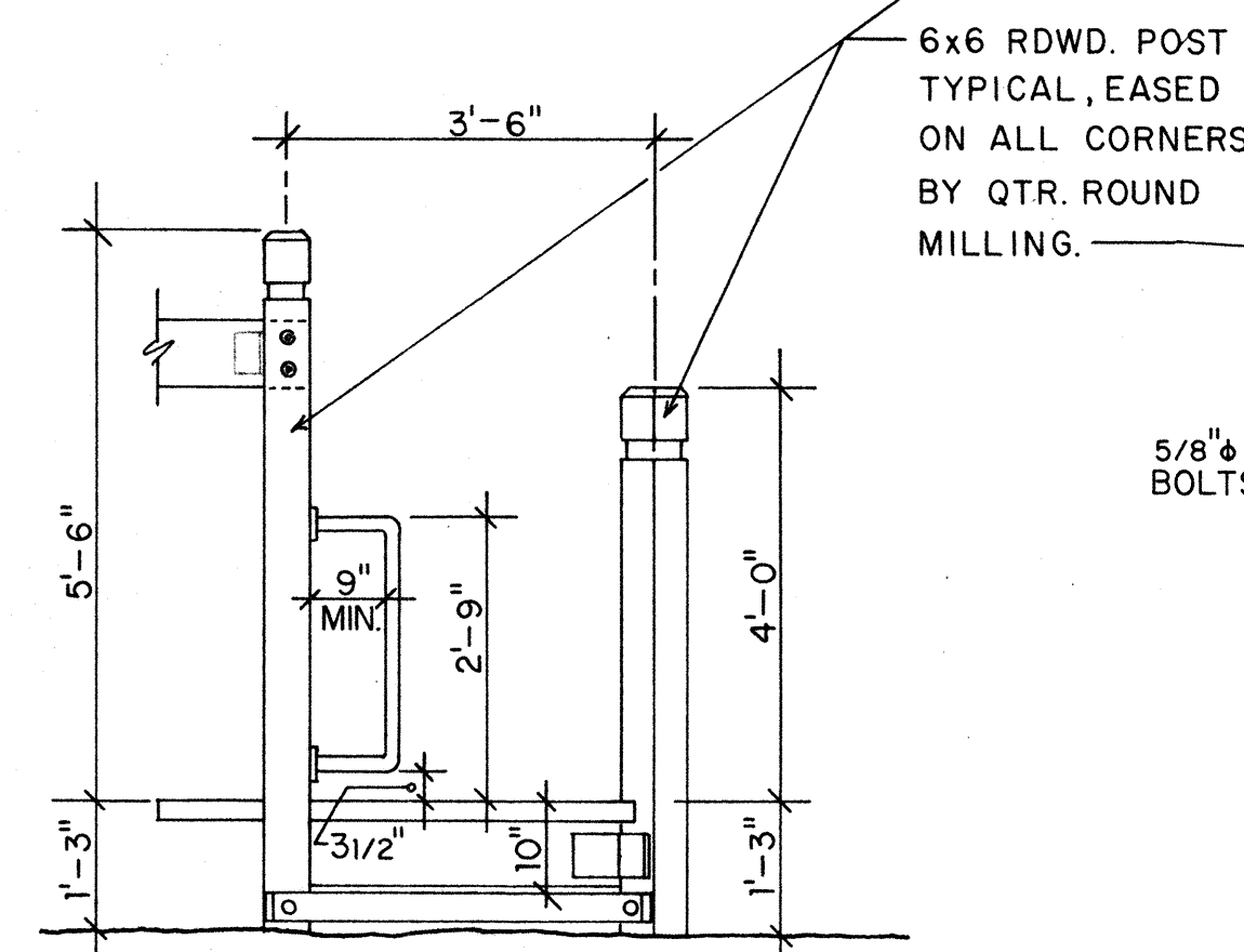
ELEVATION 5
