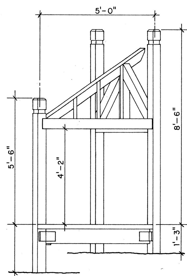
ELEVATION 10
