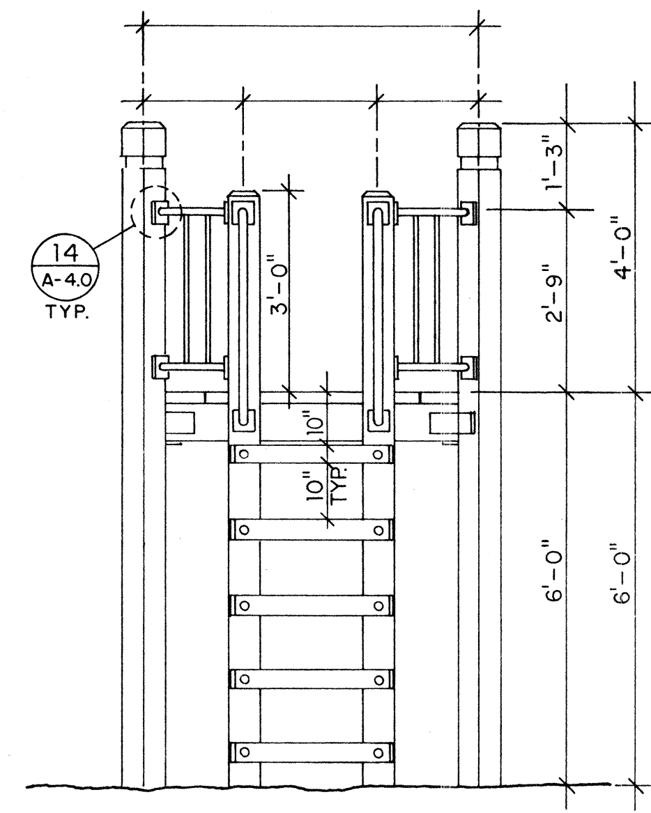
ELEVATION 3
