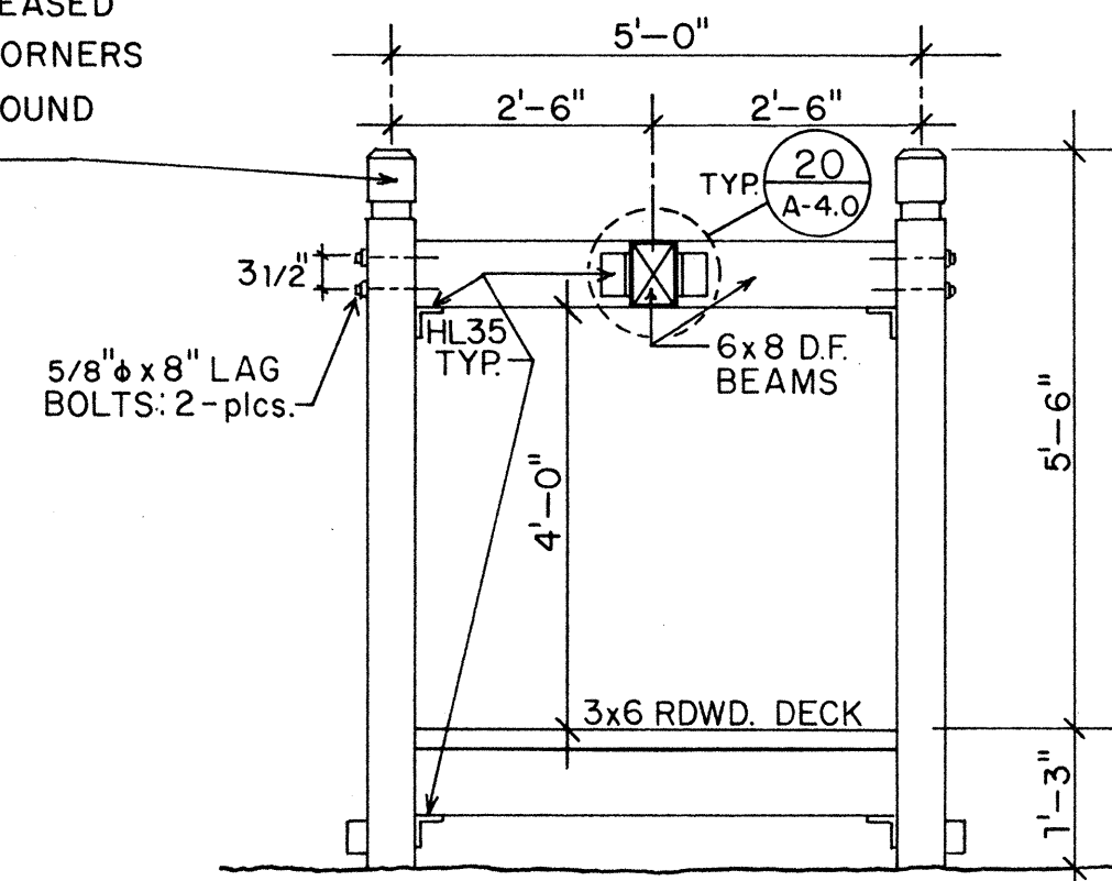
ELEVATION 6
