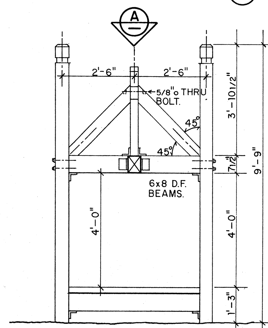
ELEVATION 5
