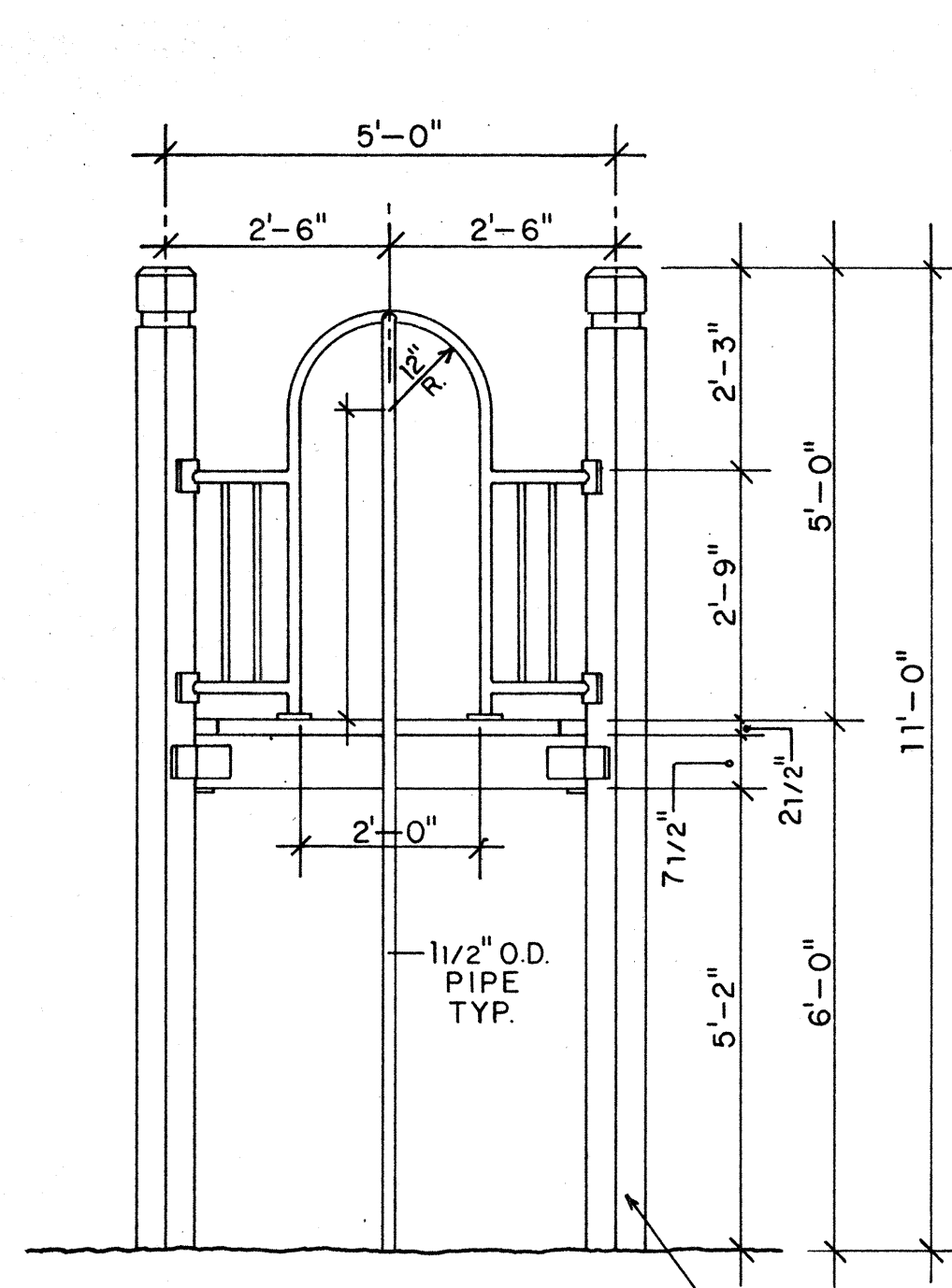
ELEVATION 1
