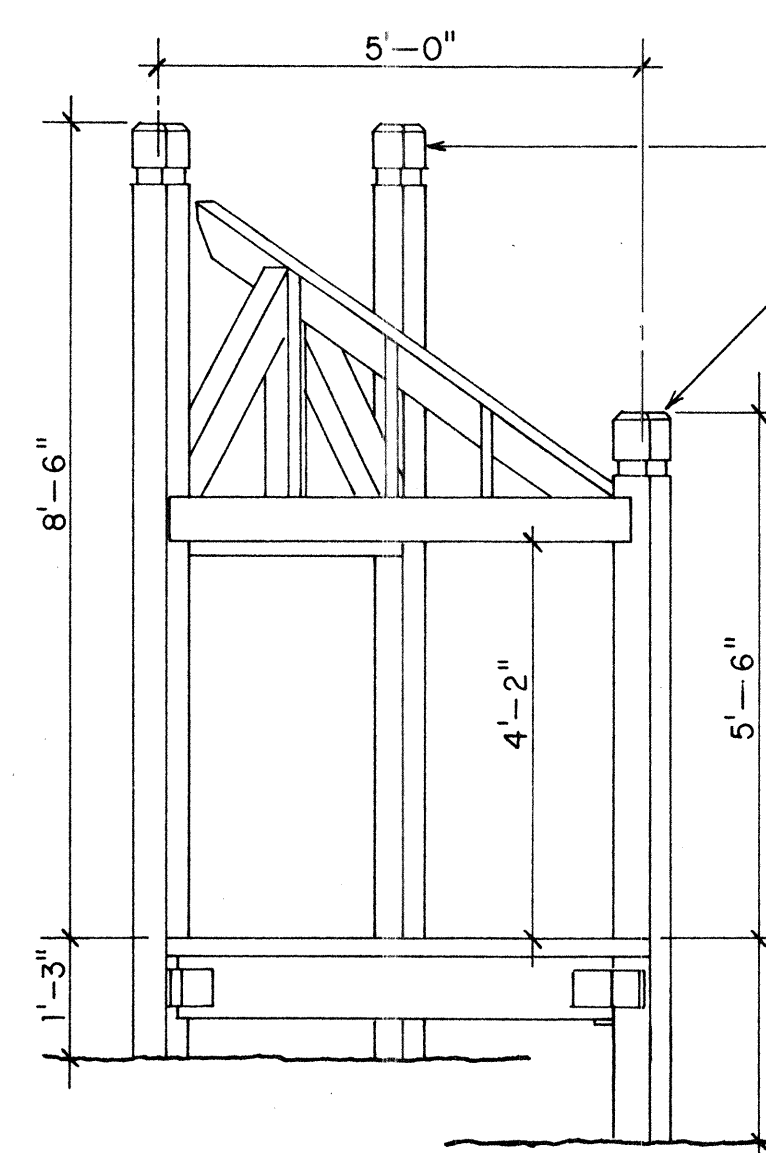
ELEVATION 12
