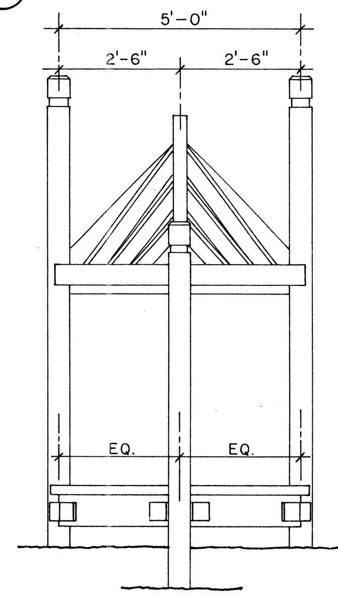
ELEVATION 11
